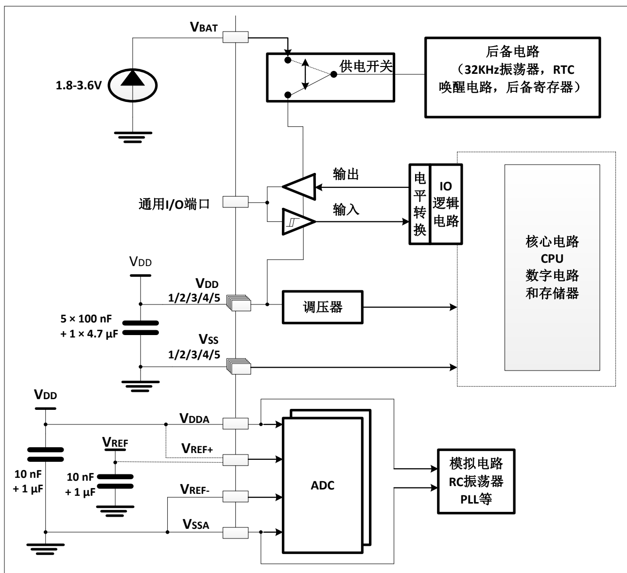
图 11 供电方案
