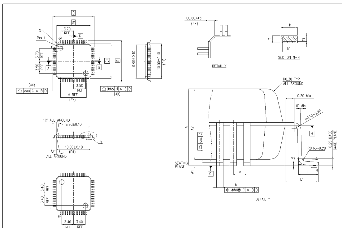
图 20 LQFP64 封装图
