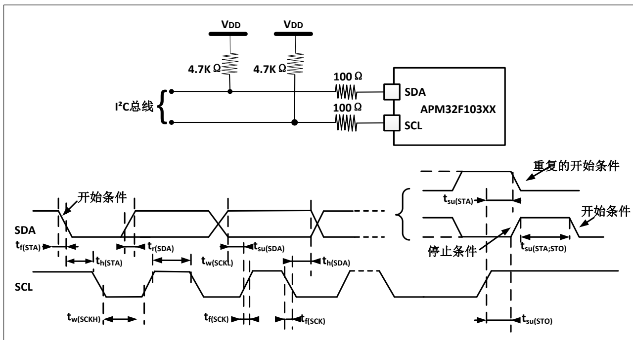
图 13 总线交流波形和测量电路 (1)
