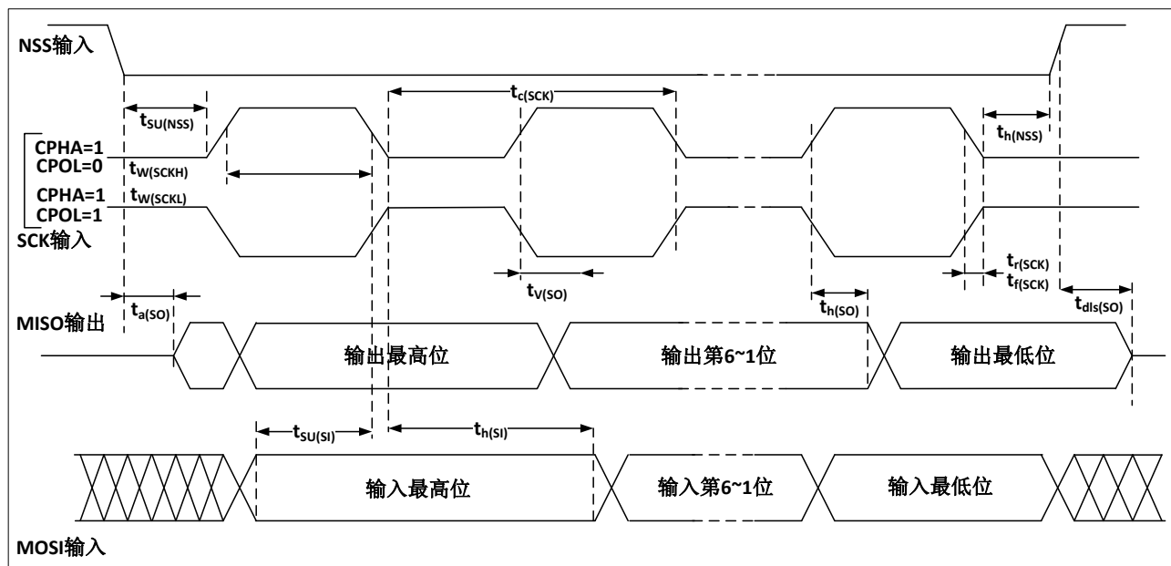
图 15 SPI 时序图 — 从模式和 CPHA=1 (1)
