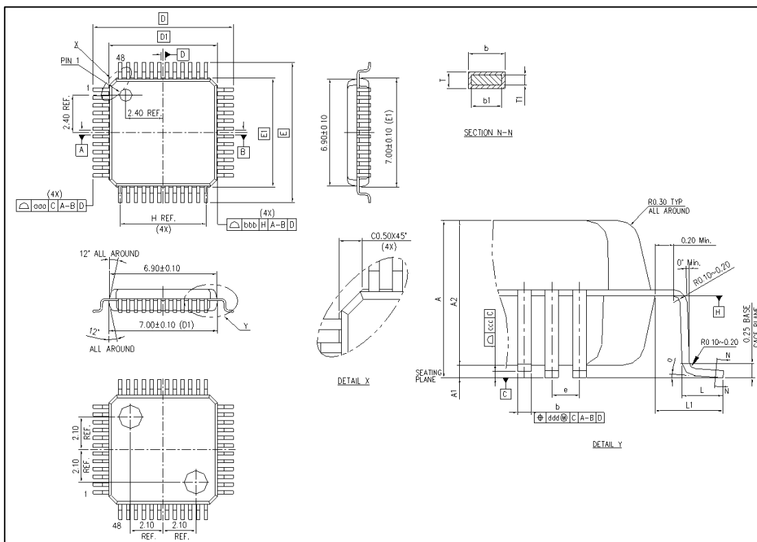
图 21 LQFP48 封装图
