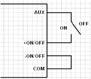
图2 遥控接线图
