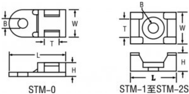
扎线扎带固定座产品工程图
