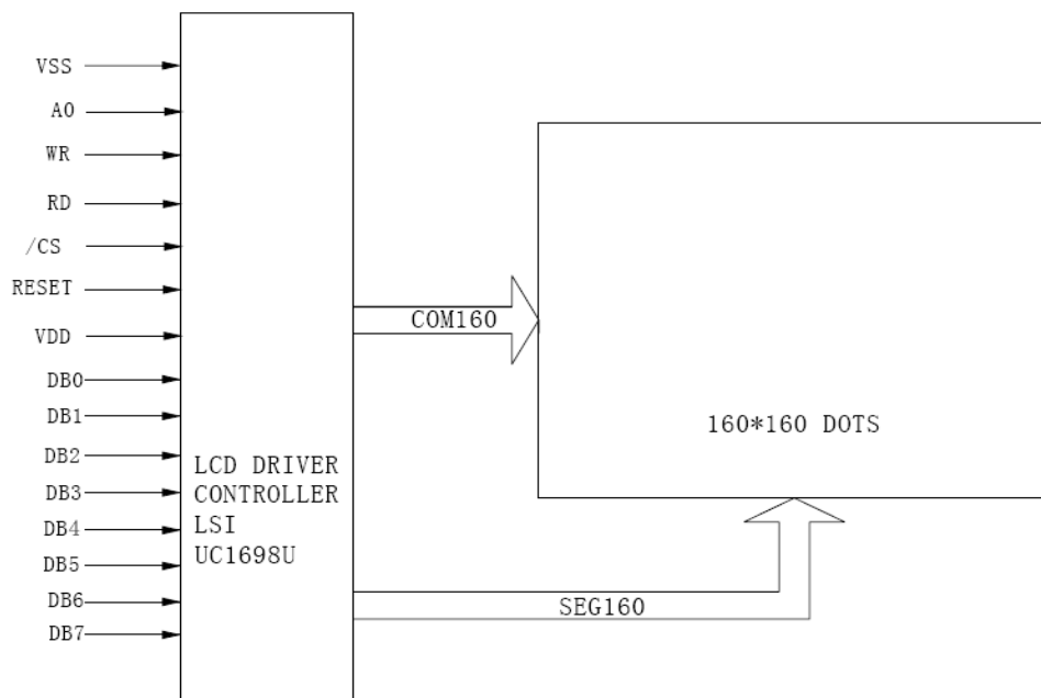
图 3.显示原理图
