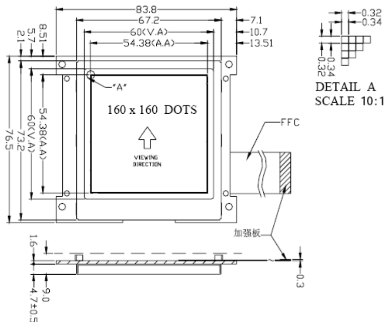
图 2.产品结构图纸
